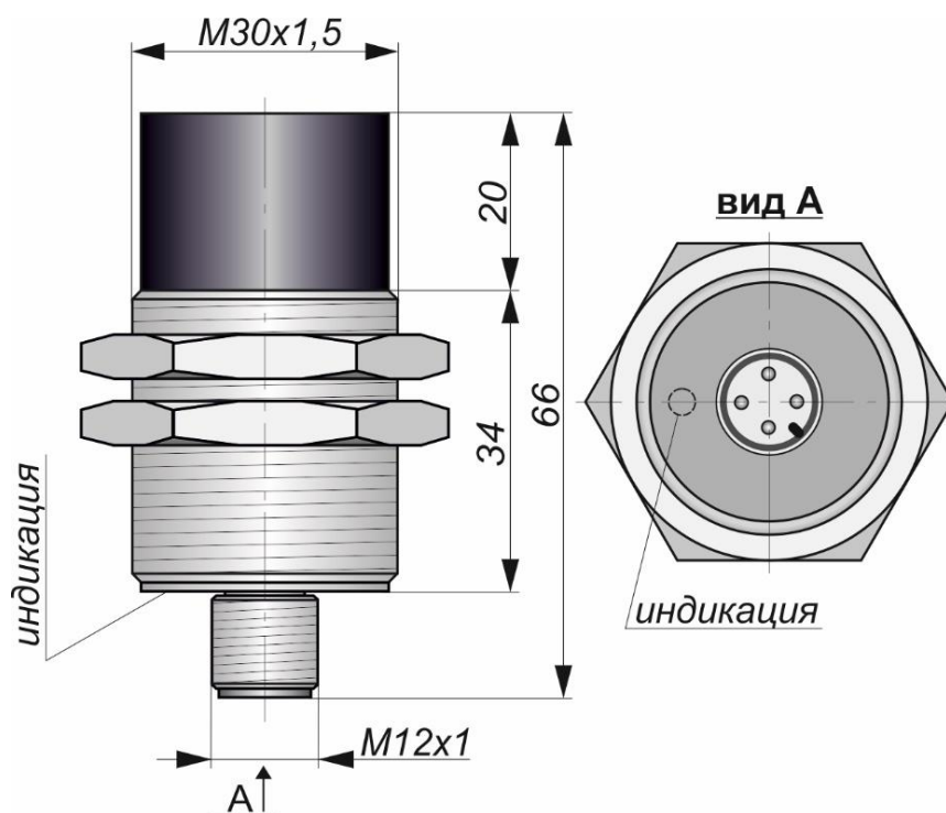
Габаритный чертеж
